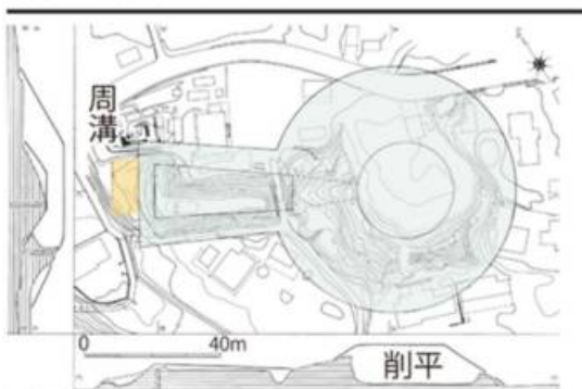
今富塚山古墳の墳丘と推定復元形（永沼1992を改変）
