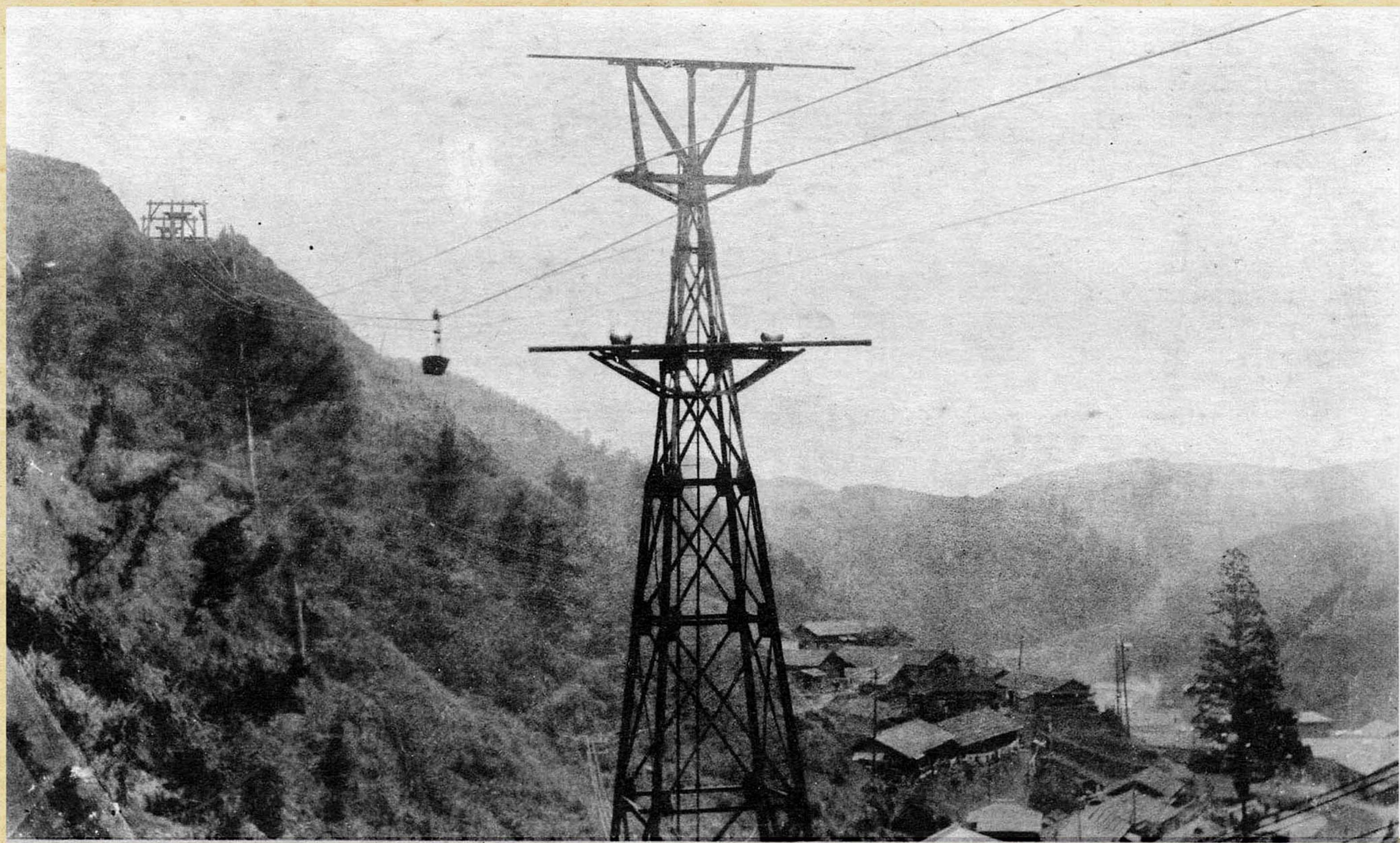
日 立 鐵 山 本 山 鐵 索 運 搬 機
