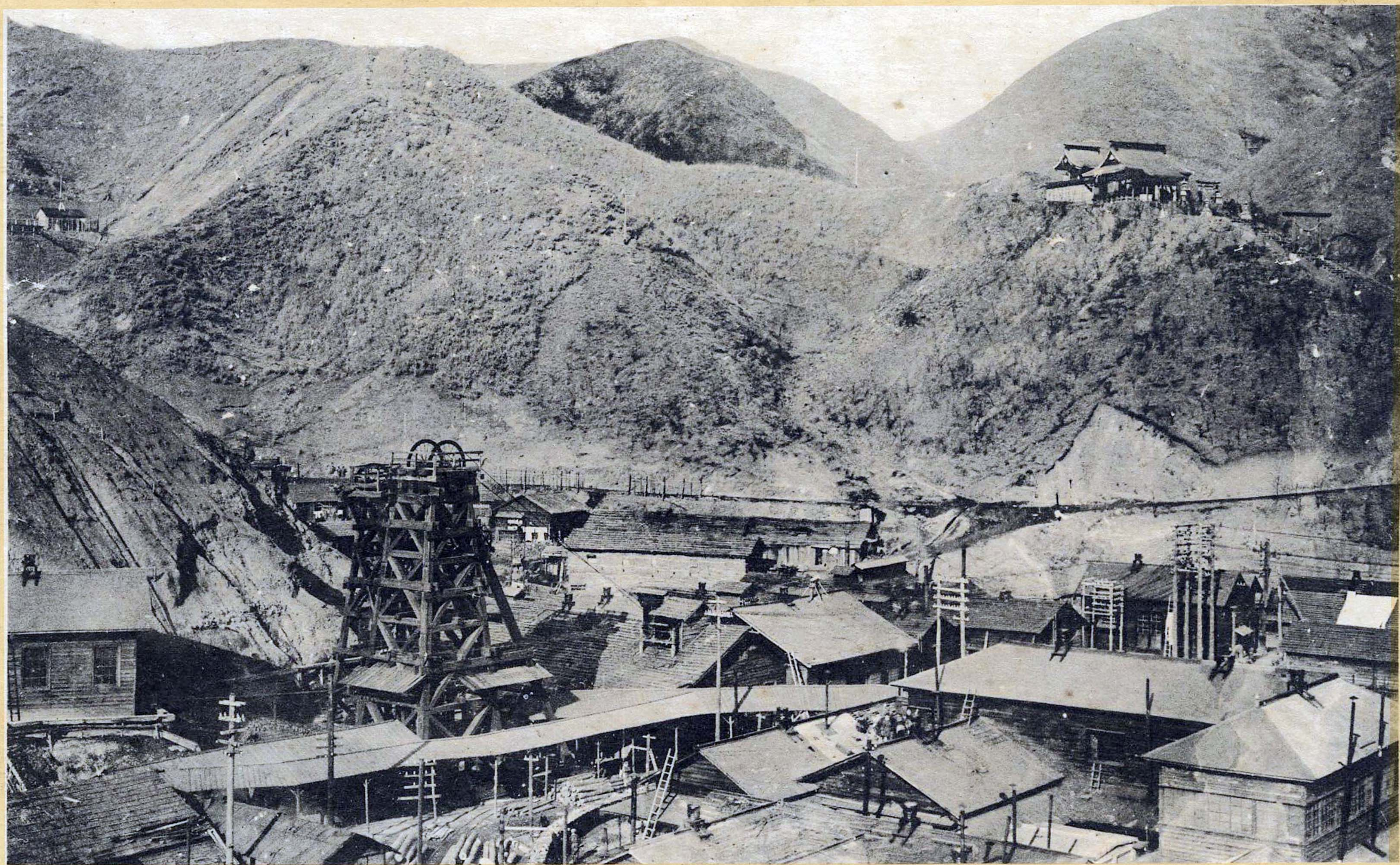
日 立 鑛 山 本 山 捲 上 機
