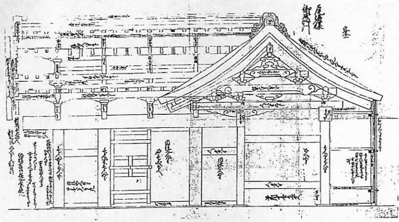
第189回 尾州邸御成門建地割 (東京国立博物館所蔵)
